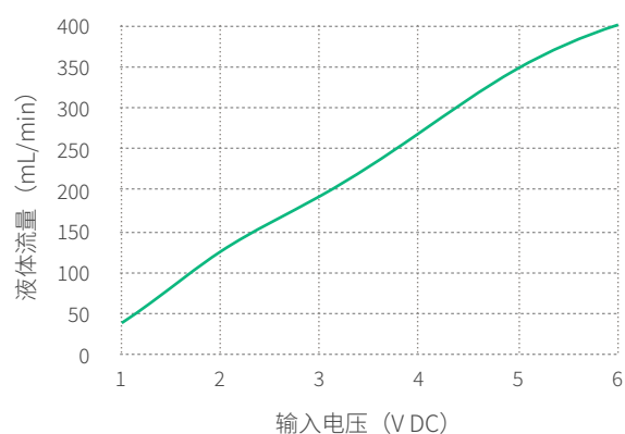
S09S配置有刷电机 电压-流量曲线
