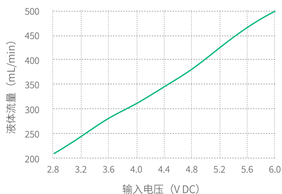
S09M配置空心杯无刷电机 电压-流量曲线
