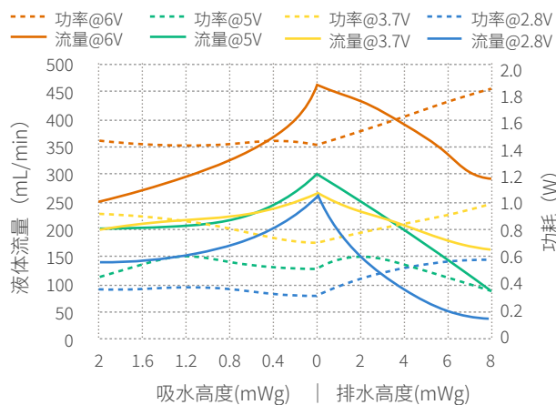
S09M 配置空心杯无刷电机 压力流量功耗曲线
