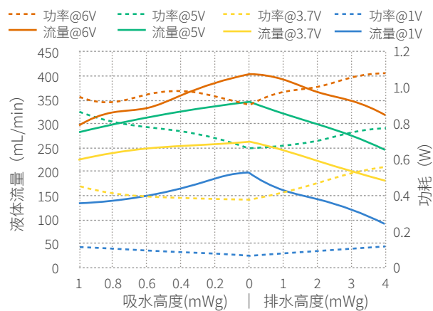
S09S 配置DC有刷电机 压力流量功耗曲线
