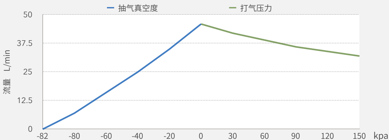
D55L 压力-流量曲线
