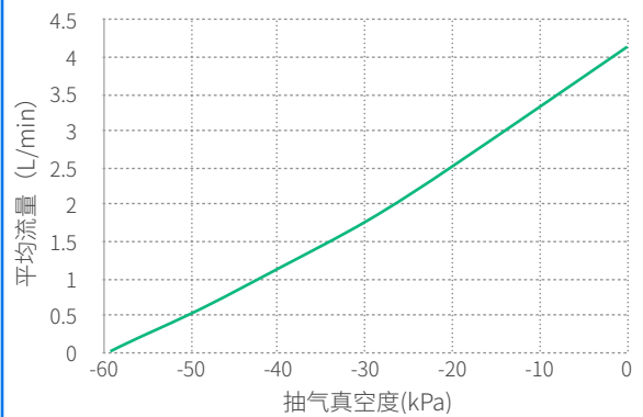
VLK4506A-24V参数曲线
