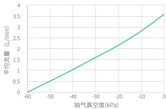
VLK4506A-12V参数曲线
