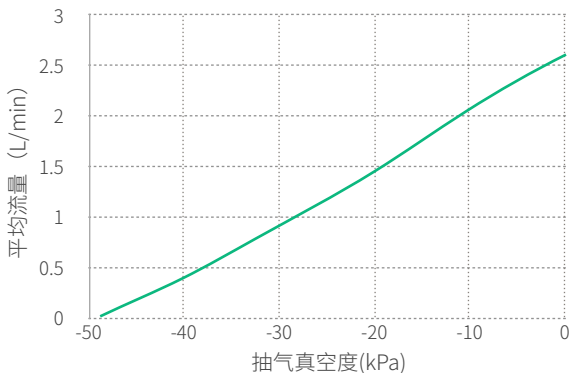
VLK5504A-12V参数曲线
