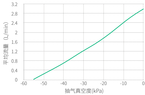
VLK5005A-12V参数曲线
