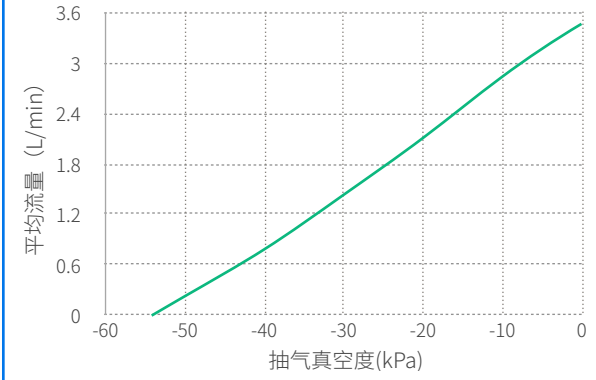
VLK5005A-24V参数曲线
