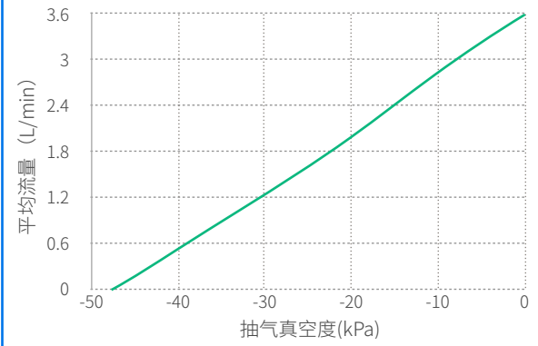
VLK5504A-12V参数曲线
